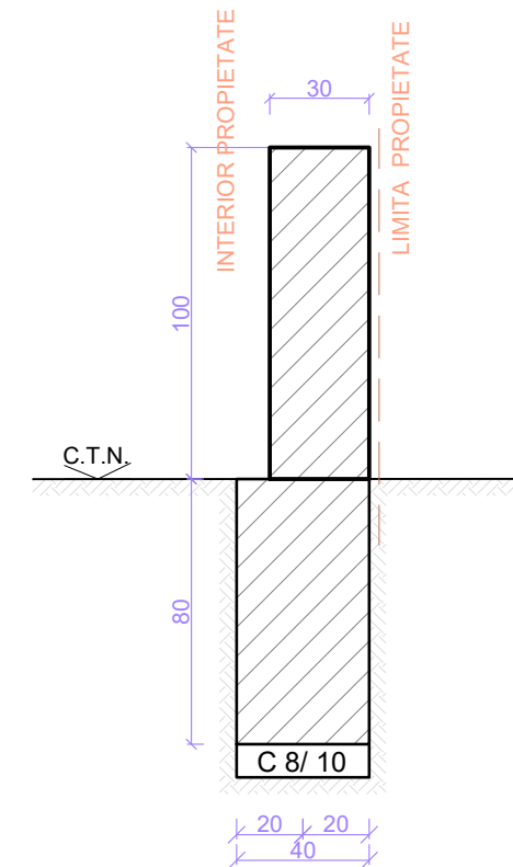
Sectiune transversala
