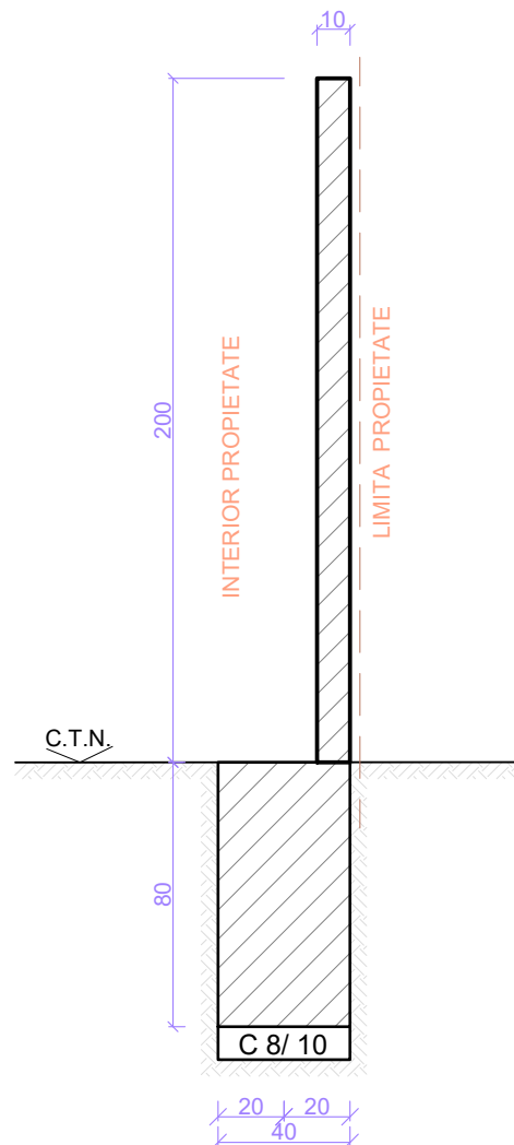
Sectiune transversala
