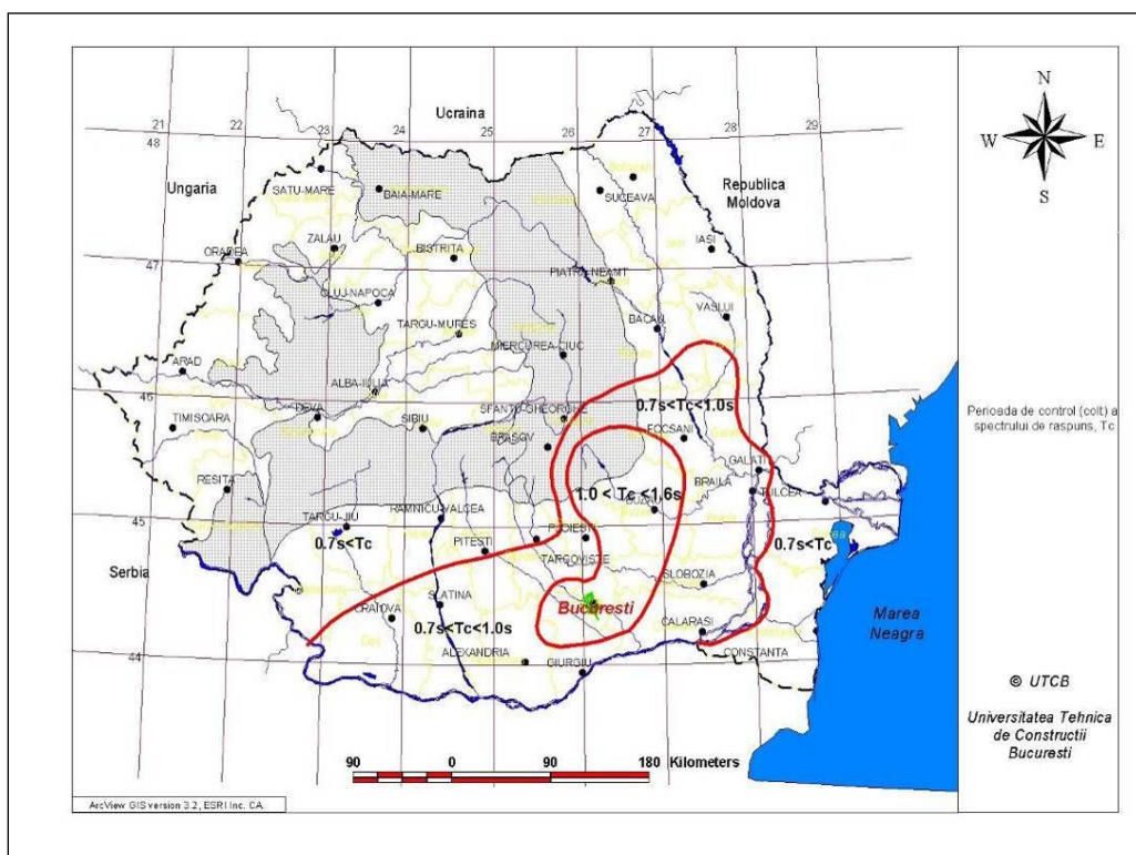
Figura 2. Zonarea teritoriului Romaniei în termeni de perioadă de control (colț), T_C a spectrului de raspuns.
