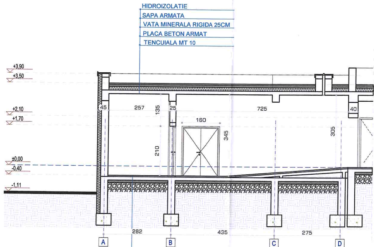
SECTIUNE A-A
